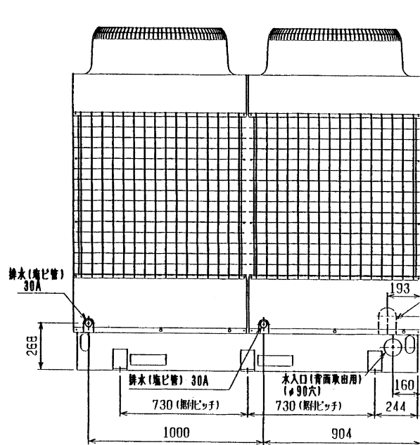
背面図
