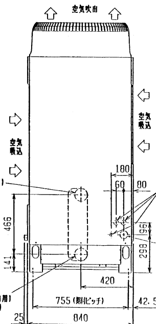
左側面図
