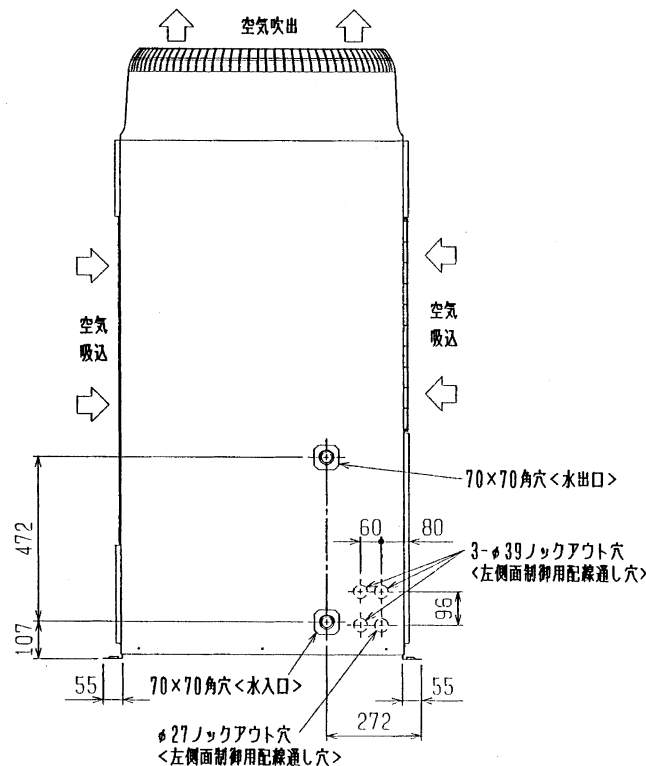
左側面図
