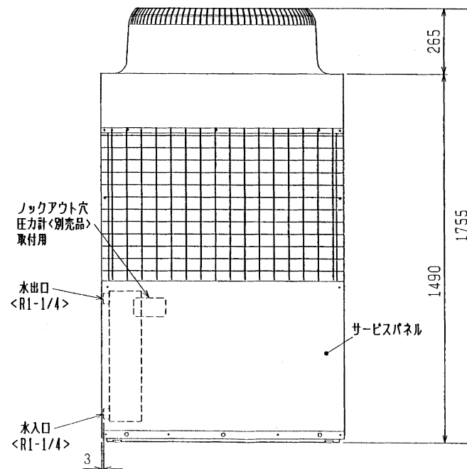
正面図
