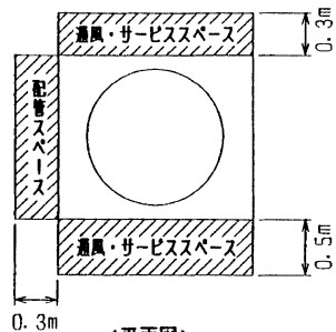
〈平面図〉 サービススペース
