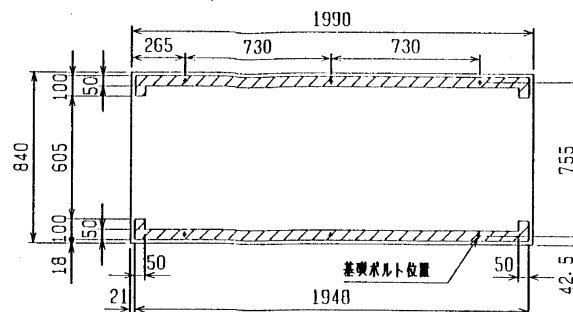
ユニット底面寸法図
