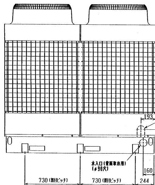
背面図
