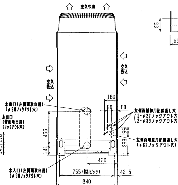
左側面図
