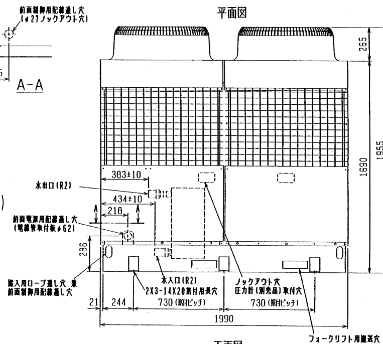
正面図
