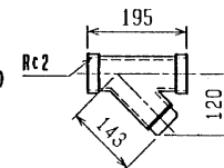
ユニット底面寸法図
