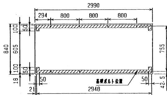
ユニット底面寸法図
