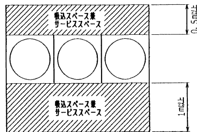
サービススペース
