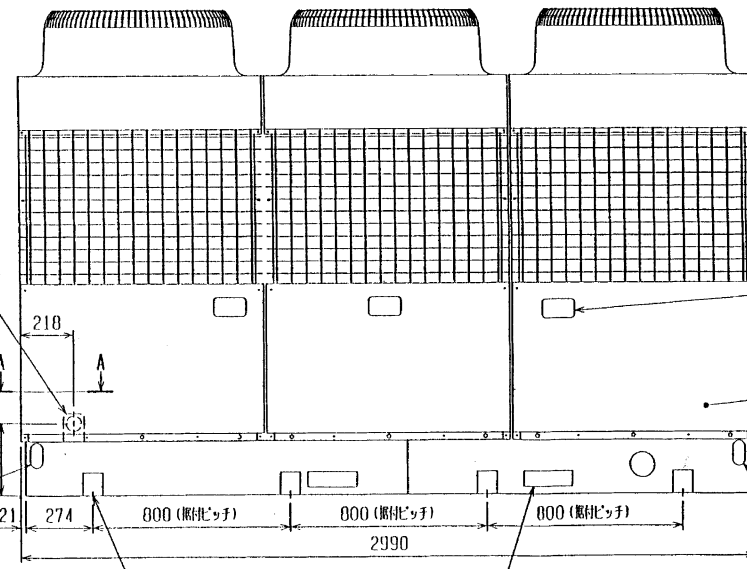
正面図
