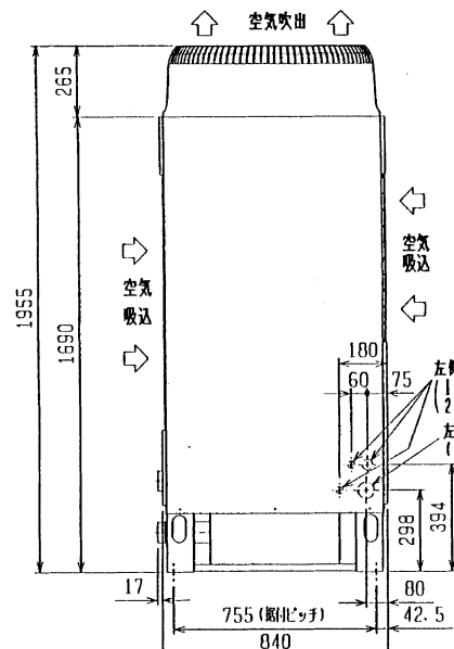
左側面図
