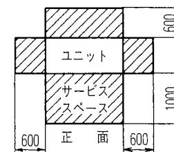
据付スペース
