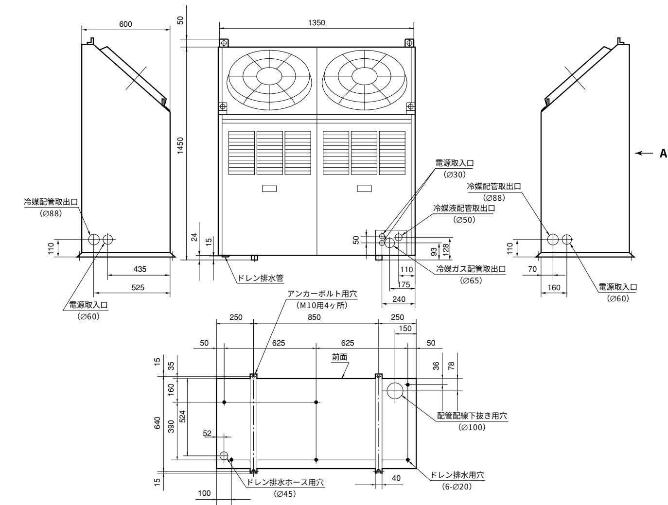
付属冷媒配管接続後の寸法 (平面図)
