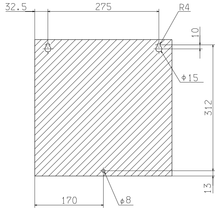
リモートコントローラ取付穴寸法
