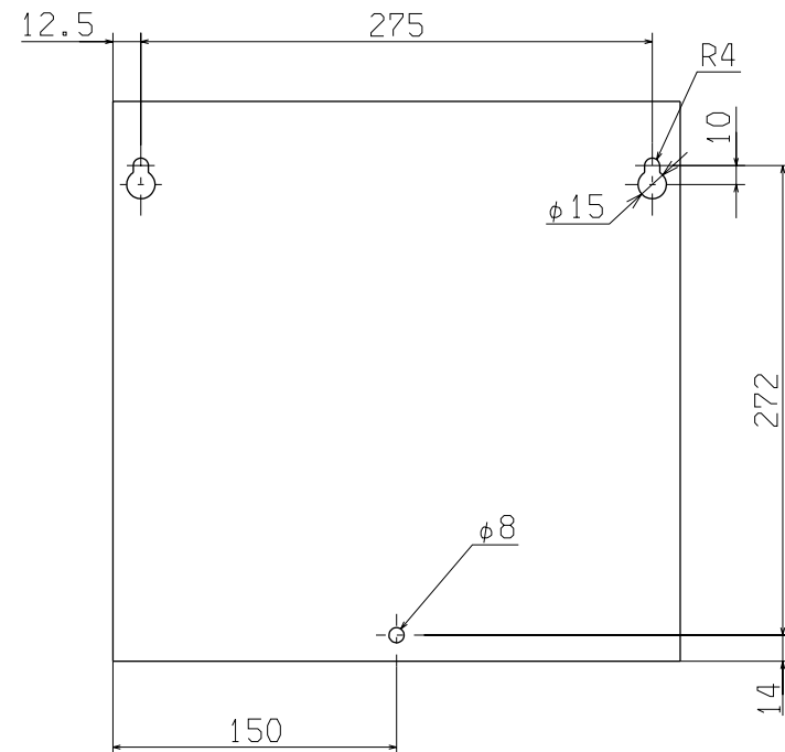
コントロールボックス取付穴寸法
