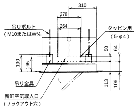
A視(新鮮空気取入口)
