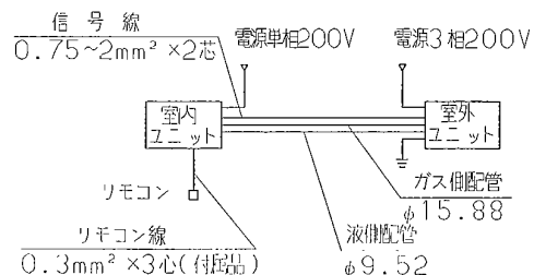
配管配線接続図
