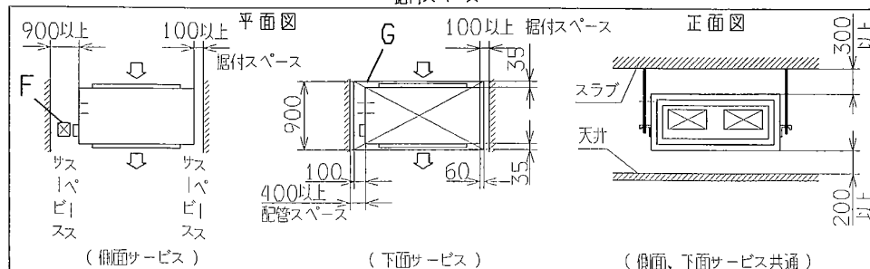
据付スペース
