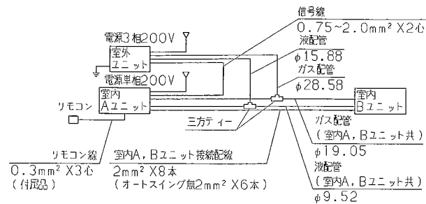
配管配線接続図
