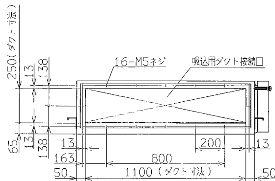
据付スペース
