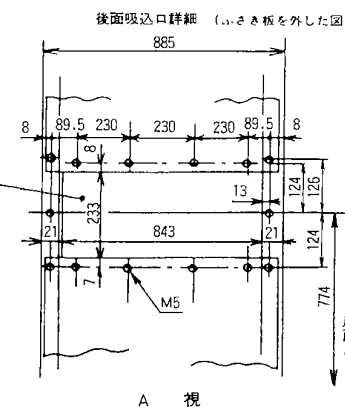
A 視
