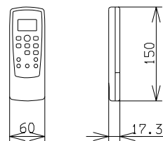
外形図（リモコン）
