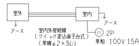
配線接続図
