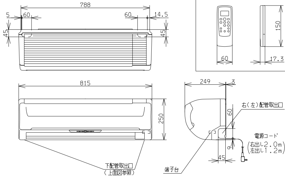
外形図（室内ユニット）
