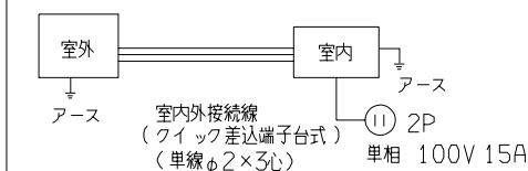
配線接続図
