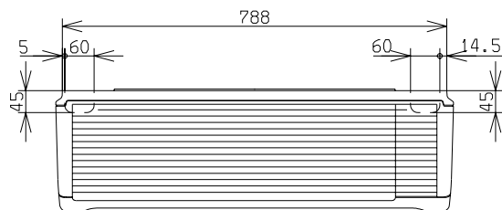
外形図(室内ユニット)
