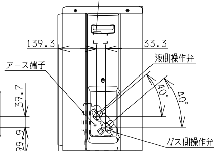
端子台
