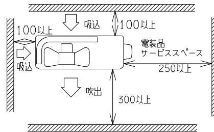
ベランダ吊りの場合
