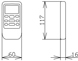
外形図(リモコン)
