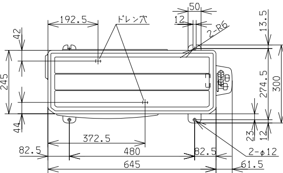
外形図( 室外ユニット )
