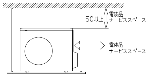
ベランダ吊りの場合
