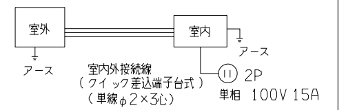
配線接続図
