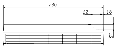
外形図(室内ユニット)
