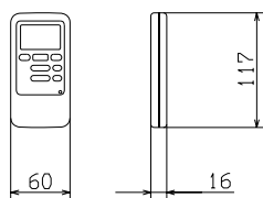
外形図(リモコン)
