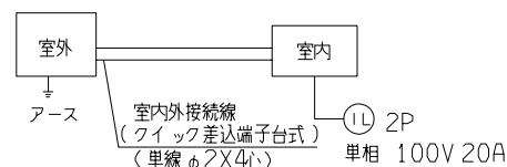
配線接続図
