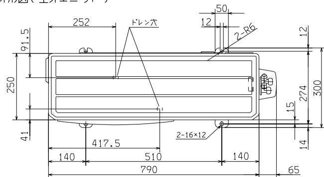
外形図(室外ユニット)
