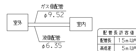
配管接続図(フレア接続)
