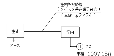
配線接続図
