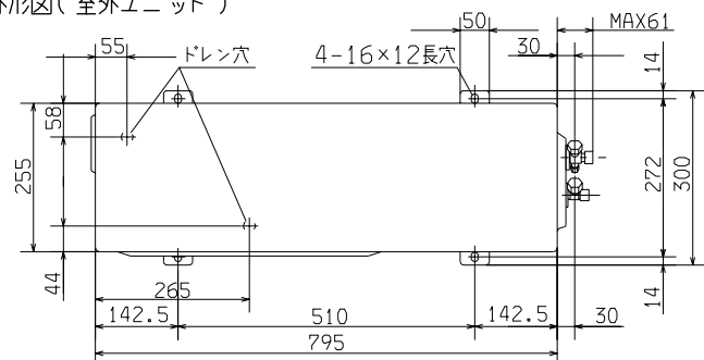
外形図(室外ユニット)
