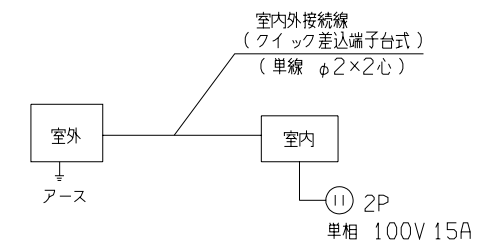
配線接続図
