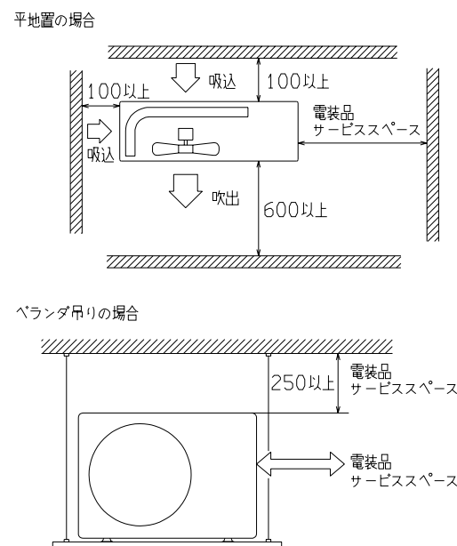
据付スペース(室外ユニット)
