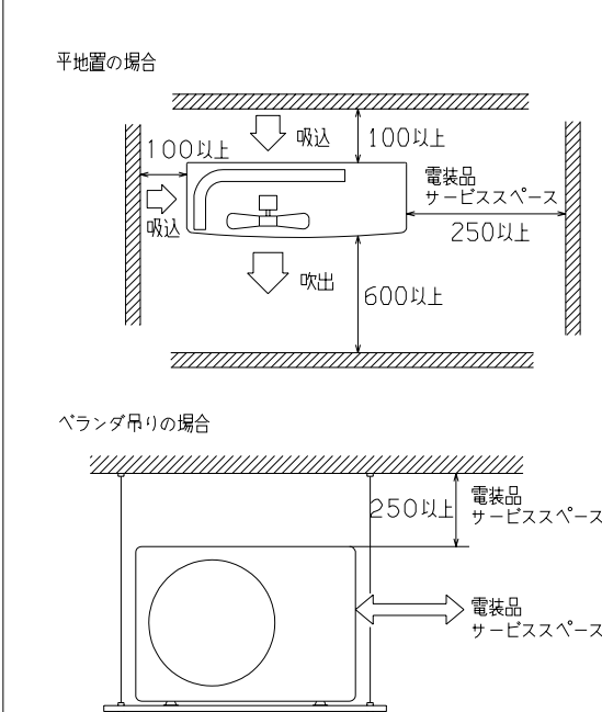
据付スペース(室外ユニット)
