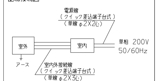
配線接続図
