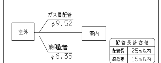
配管接続図(フレア接続)
