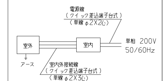
配線接続図 注1)アースは必ず取ってください。
