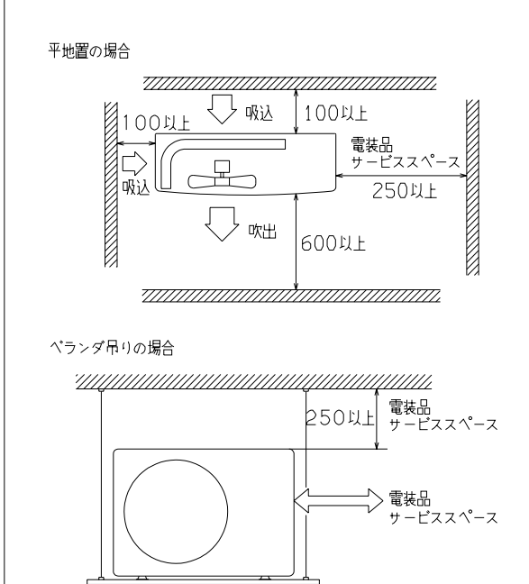
据付スペース(室外ユニット)
