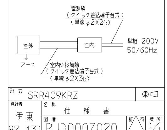
配線接続図
