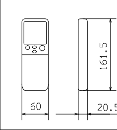
外形図(リモコン)
