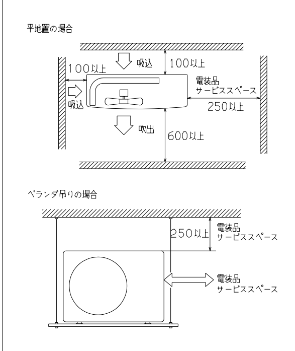
据付スペース(室外ユニット)
