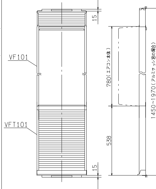
テラス窓用据付枠 (部品形名:VFT101) 別売部品
