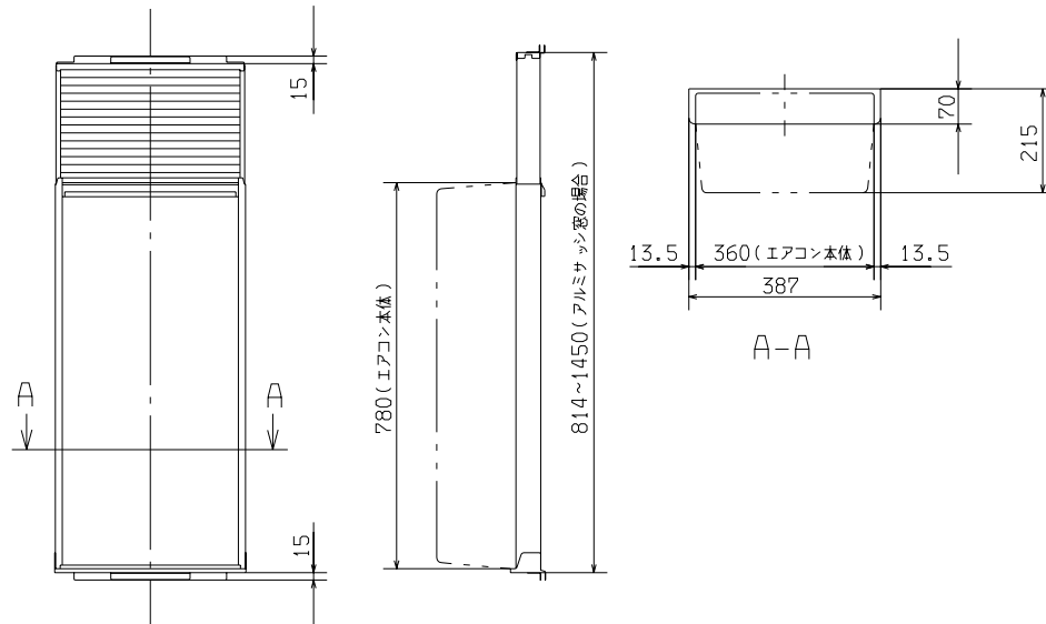
標準据付枠 (部品形名:VF101) 付属部品
