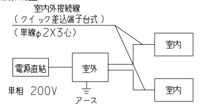
配線接続図
