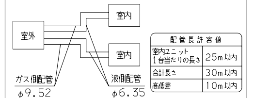
配管接続図(フレア接続)
