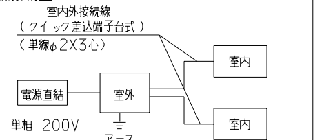
配線接続図
