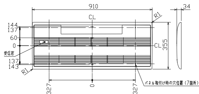
化粧パネル外形図 (TIP25-W,C)
