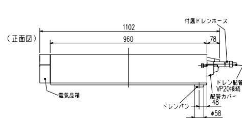
化粧パネル外形図 (TP26-W/C)
