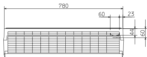
外形図(室内ユニット)
