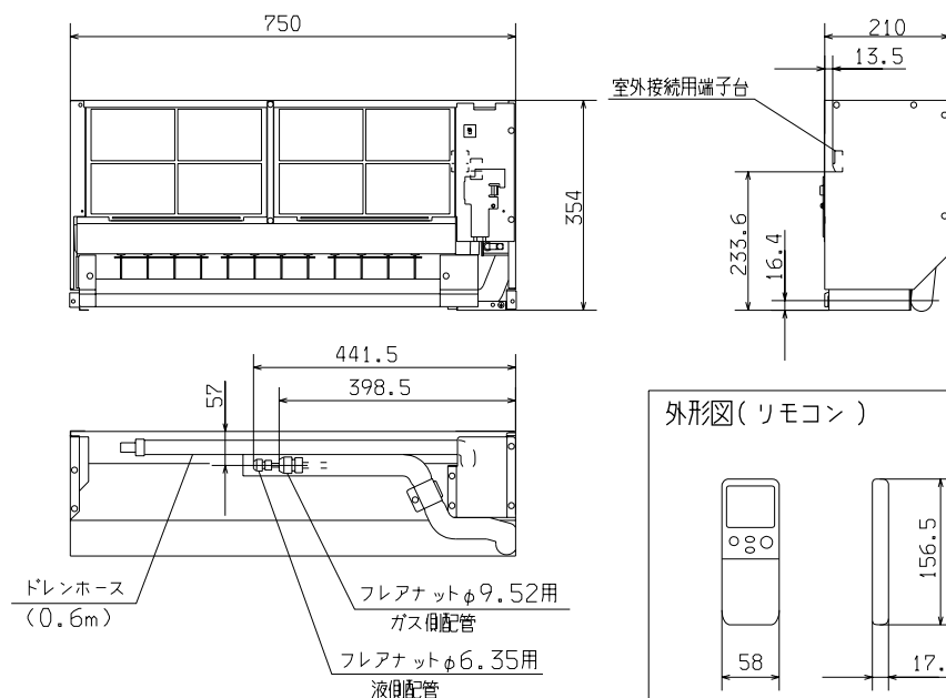
外形図(室内ユニット)
