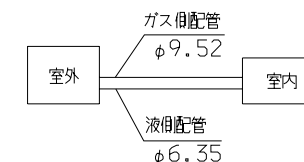
配管接続図(フレア接続)
