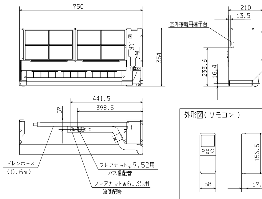
外形図(室内ユニット)
