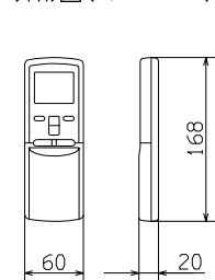
外形図(リモコン)
