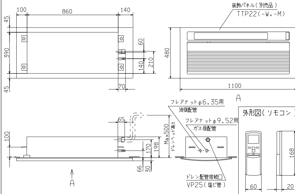
外形図(室内ユニット)
