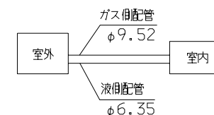
配線接続図
