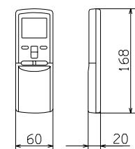
外形図(リモコン)
