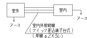
配線接続図 注1)アースは室内、室外いずれかで必ず取ってください。
