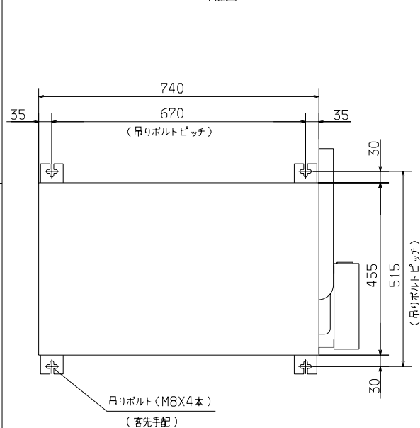
据付寸法(室内ユニット) 平面図
