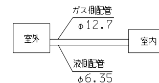
配管接続図(フレア接続)
