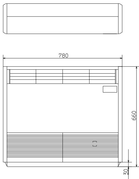
外形図(室内ユニット)
