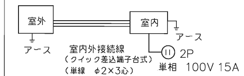
配線接続図
