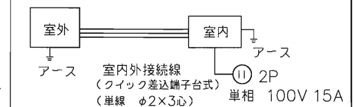
配線接続図
