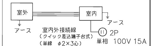
配線接続図
