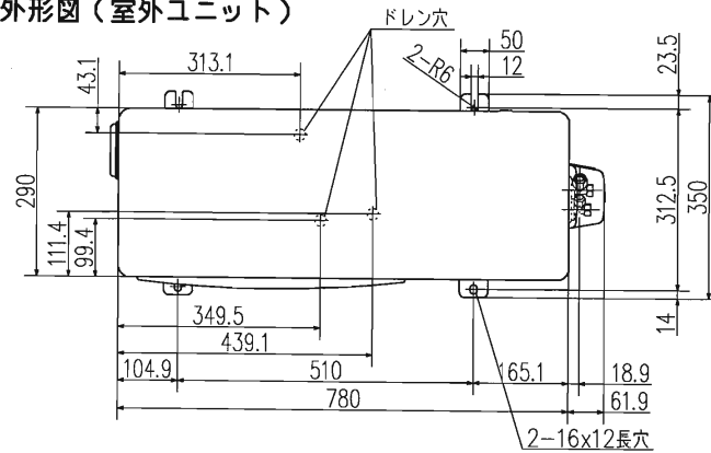
外形図（室外ユニット）
