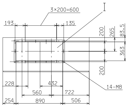
吹出口(送風機室天井)
