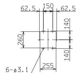
Z部 吸込口兼外気取入口(側面)
