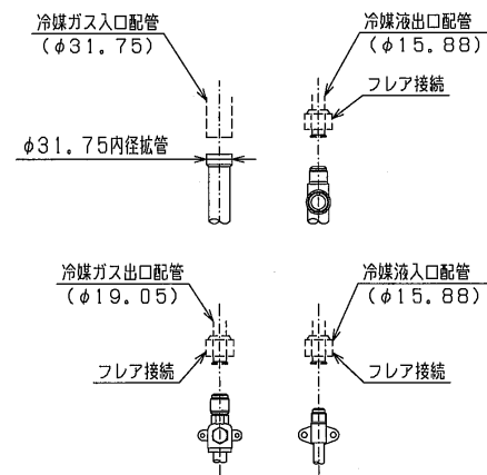
配管接続部詳細
