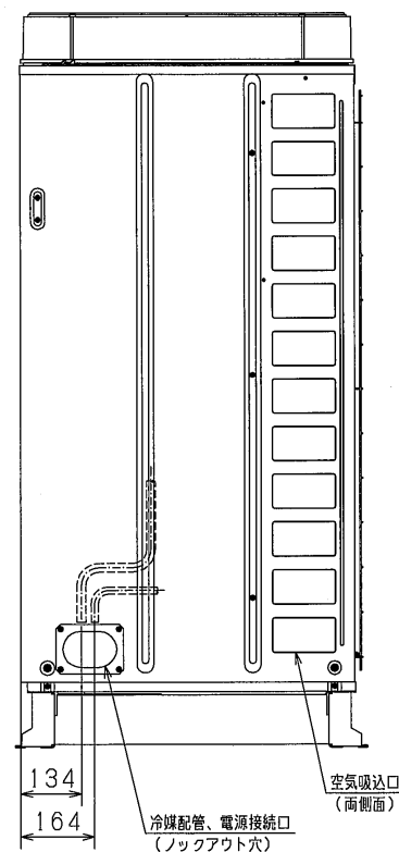
HRC55A1 側面図
