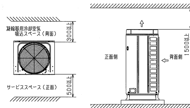
サービススペース
