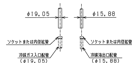
配管接続部詳細
