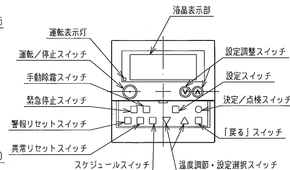
機器配置図
