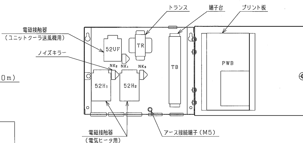
機器配置図
