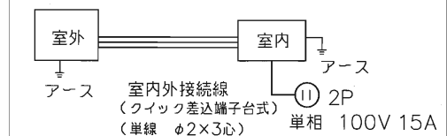
配線接続図
