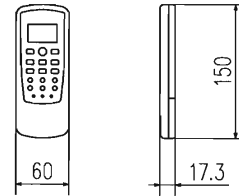
外形図（リモコン）
