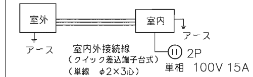
配線接続図
