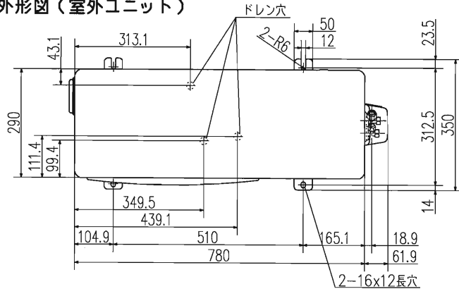
外形図（室外ユニット）
