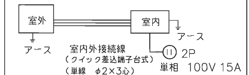
配線接続図
