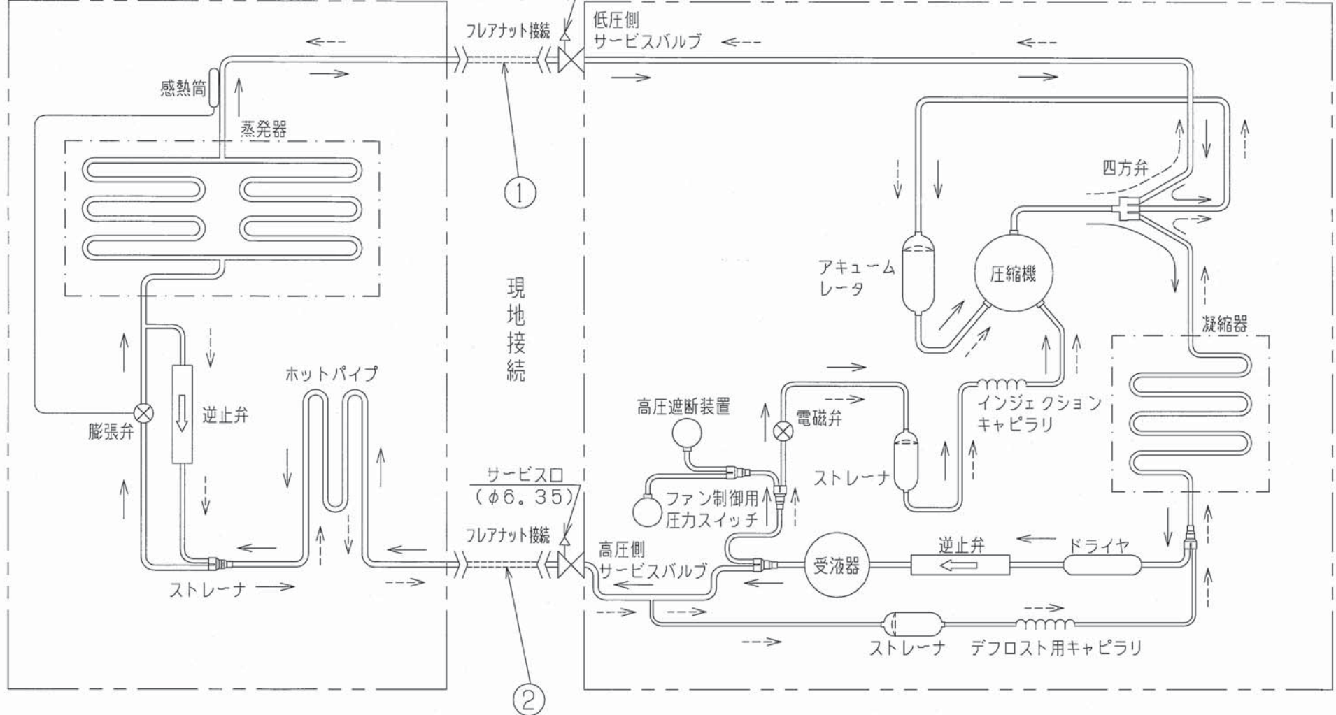
現地接続冷媒配管サイズ
