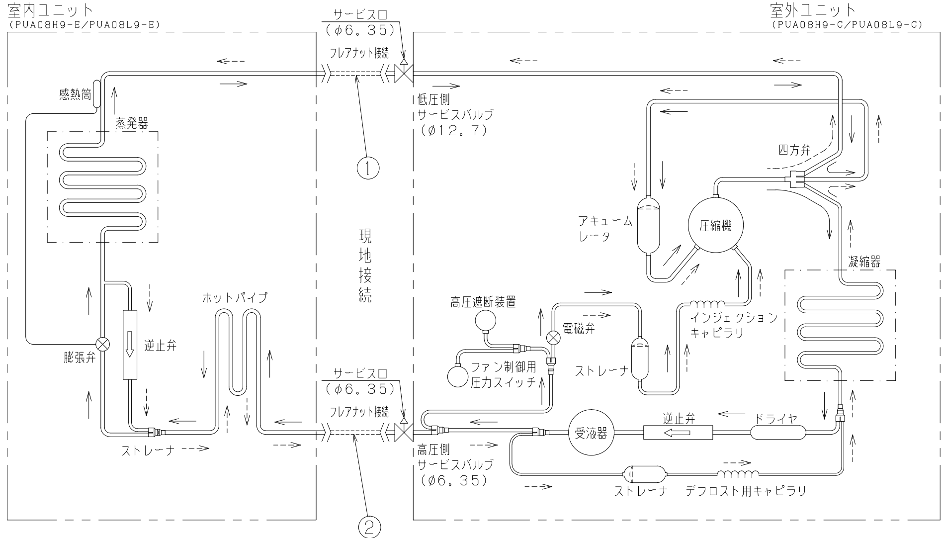
現地接続冷媒配管サイズ
