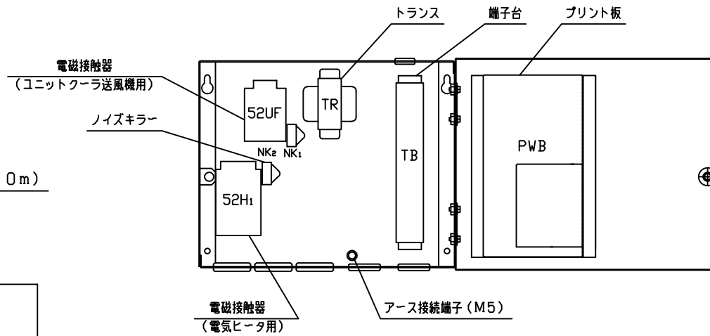
機器配置図
