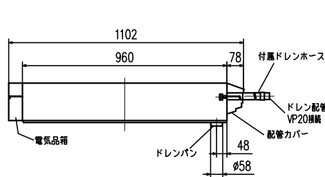
化粧パネル外形図 (ITPN-23W,23C,23M,23T)
