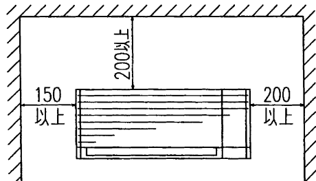
据付スペース
